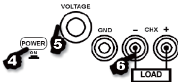
Figura 8 – Conectarea sursei la sarcina pentru modelele UTP1303 și UTP1305 sau fiecare dintre sursele de alimentare reglabile ale modelelor UTP3303 și UTP3305
