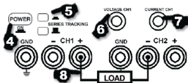
Figura 10 – Modul de funcționare în serie al surselor de alimentare reglabile ale modelelor UTP3303 și UTP3305.
